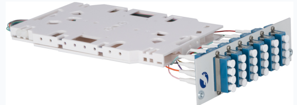
Abbildung: geöffnet, voll bestückt
